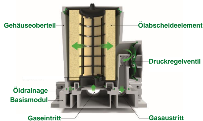
Abb. 3: ProVent 2 500 Komplettmodul im Schnitt
